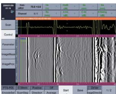
Raw TOFD Image
