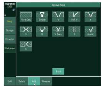
UT Flat Weld Groove
